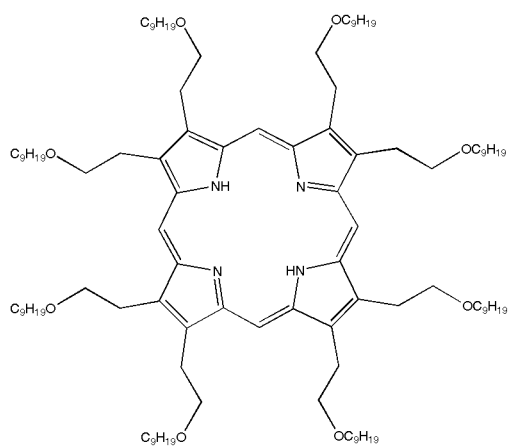
Porphyrin
