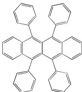
Rubrene
