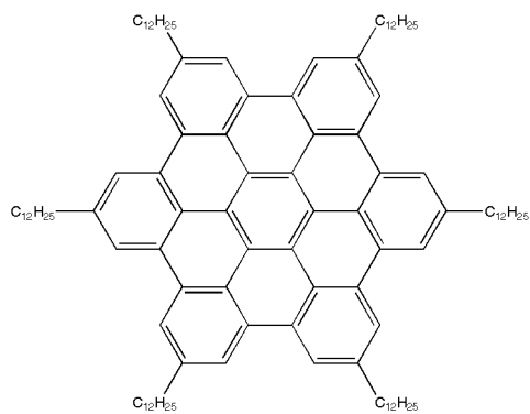
peri-Hexabenzocoronene
